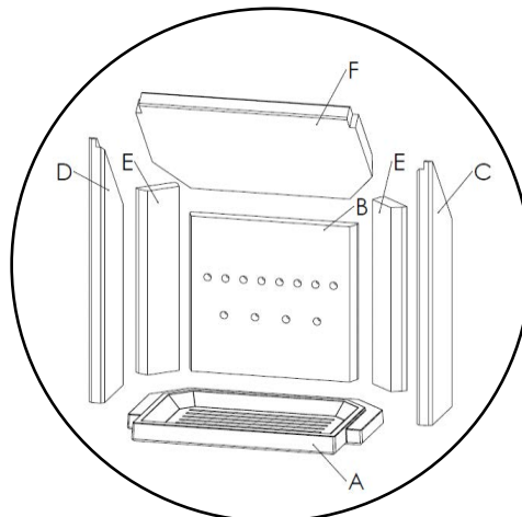
Abbildung 15 – Feuerraumauskleidung mit Rost
