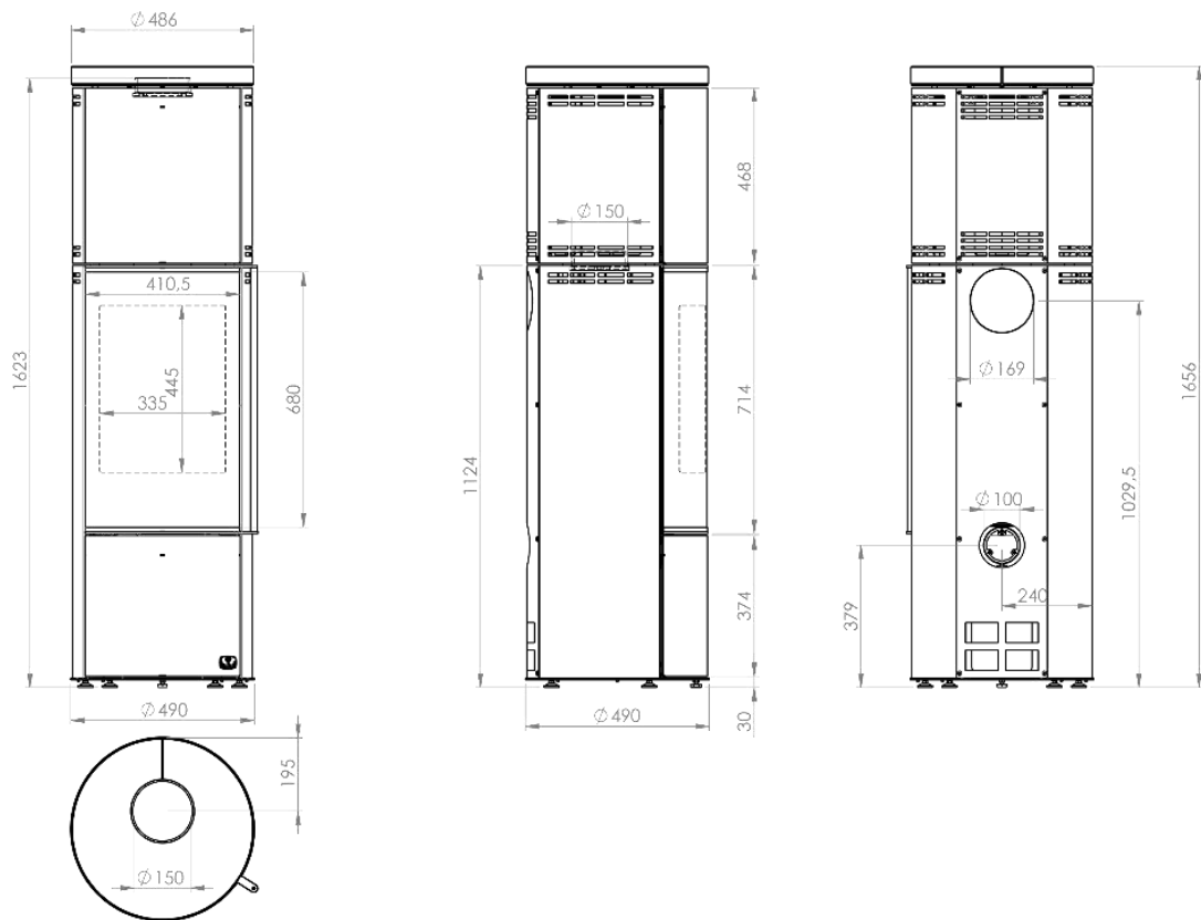
Abbildung 5 - Hauptmaße
