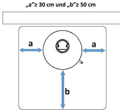
Abbildung 9 - Bodenplatte
