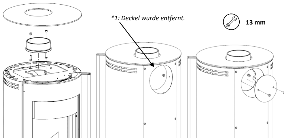
Abbildung 7 - Abgasstutzen und Abdeckung demontieren
