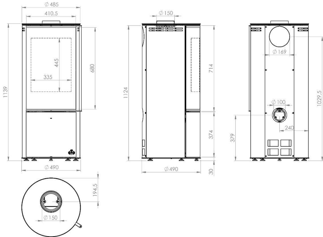
Abbildung 2 - Hauptmaße
