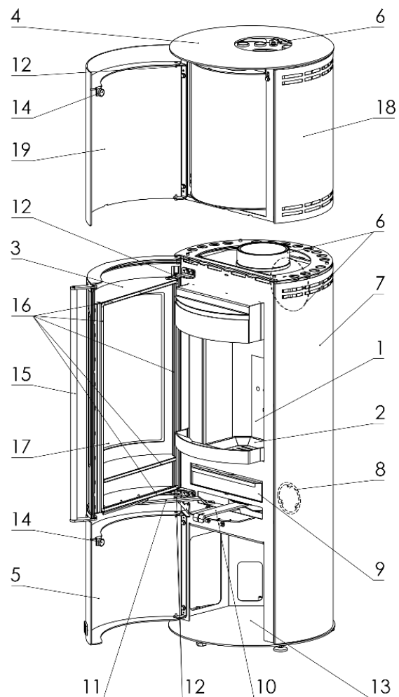
Abbildung 1 – Aufbau des Geräts
