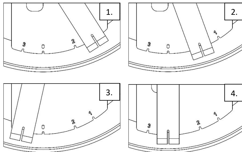
Abbildung 14 – Regelungsscheibe
