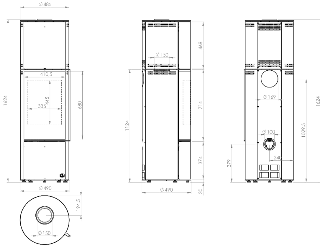
Abbildung 4 - Hauptmaße
