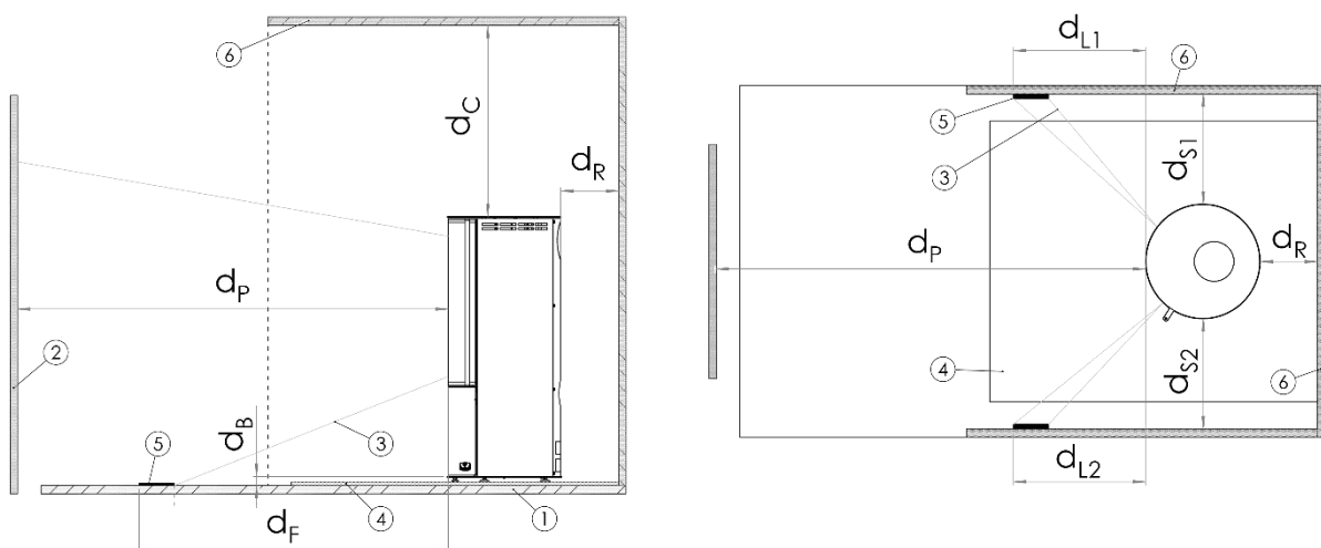
Abbildung 10 – Schematische Darstellung der Mindestabstände (siehe Tabelle 2)
