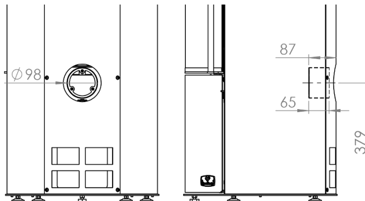
Abbildung 8 - Verbrennungsluftanschluss
