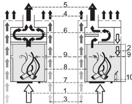
Abbildung 6 – Fire-Plus System, schematische Darstellung
