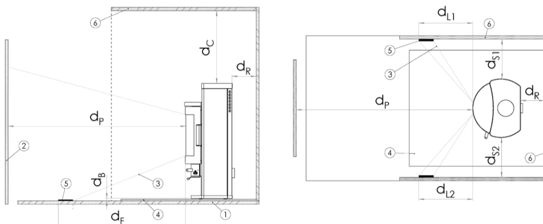
Abbildung 11 - Schematische Darstellung der Mindestabstände (siehe Tabelle 2)
