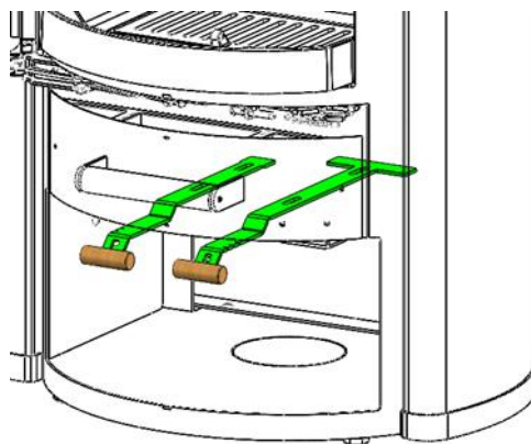
Abbildung 14 - P: Primärluftregler, S: Sekundärluftregler
