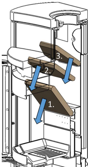
Abbildung 16 – Zugang zum Rauchraum
