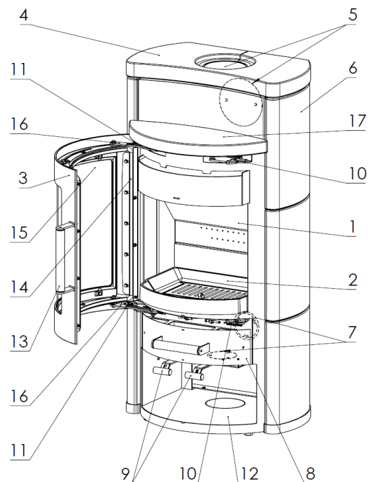
Abbildung 2 – Aufbau des Geräts
