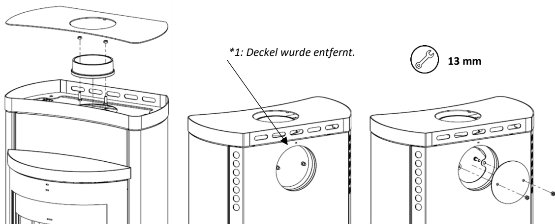
Abbildung 8 - Abgasstutzen und Abdeckung demontieren
