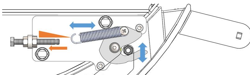
Abbildung 17 - Schnappverschluss
