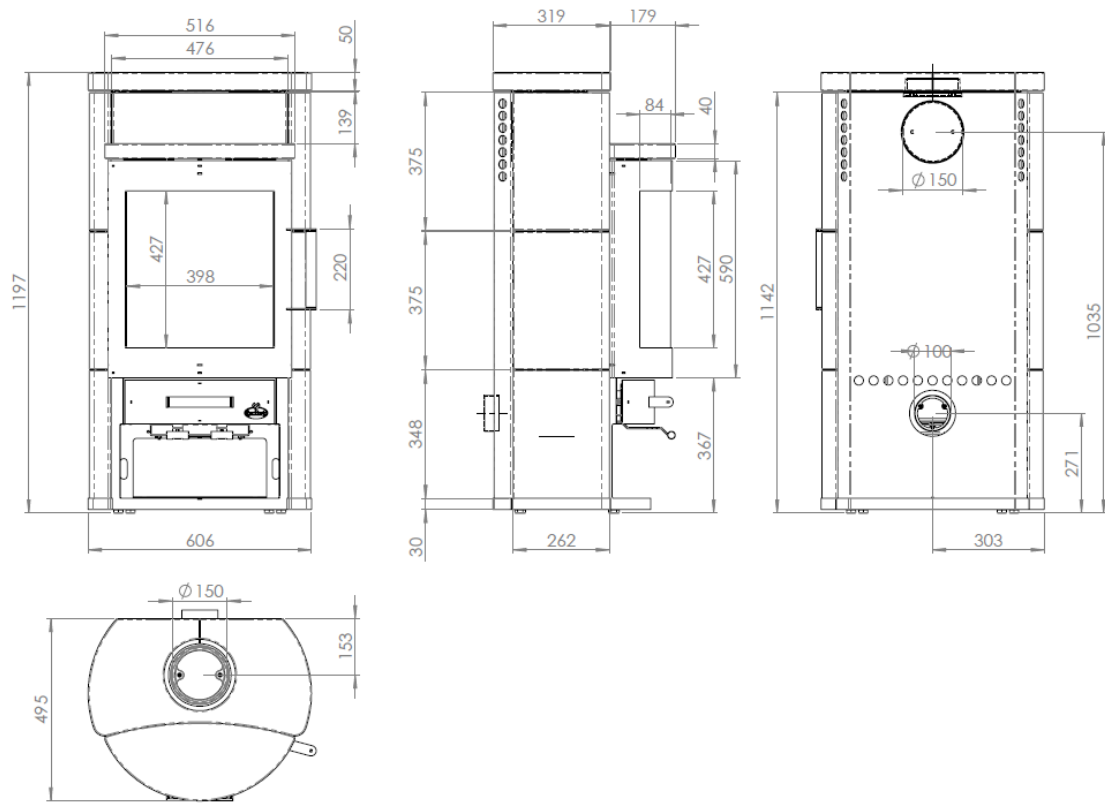
Abbildung 3 - Hauptmaße
