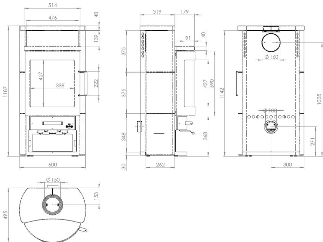
Abbildung 6 - Hauptmaße
