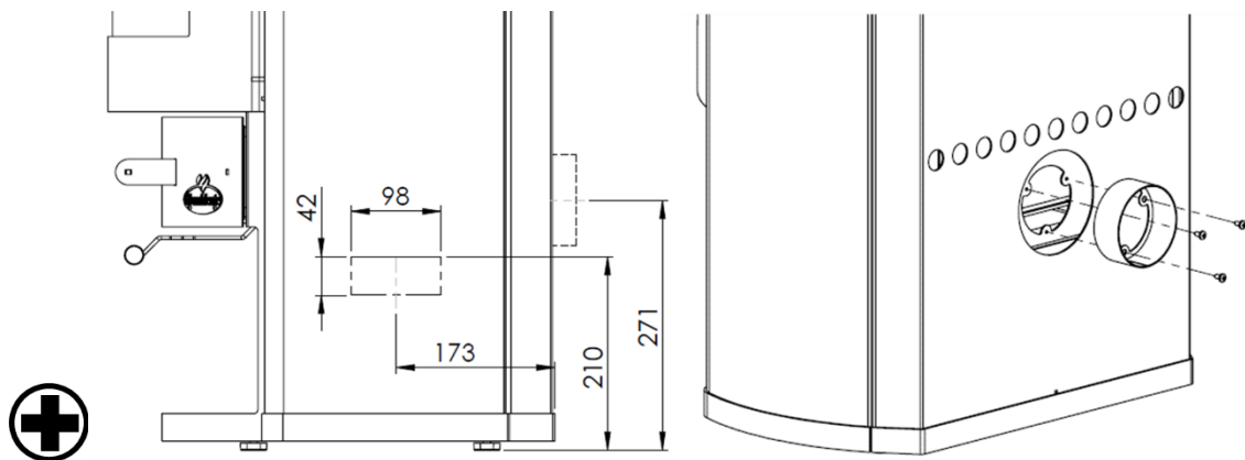
Abbildung 9 - Verbrennungsluftanschluss
