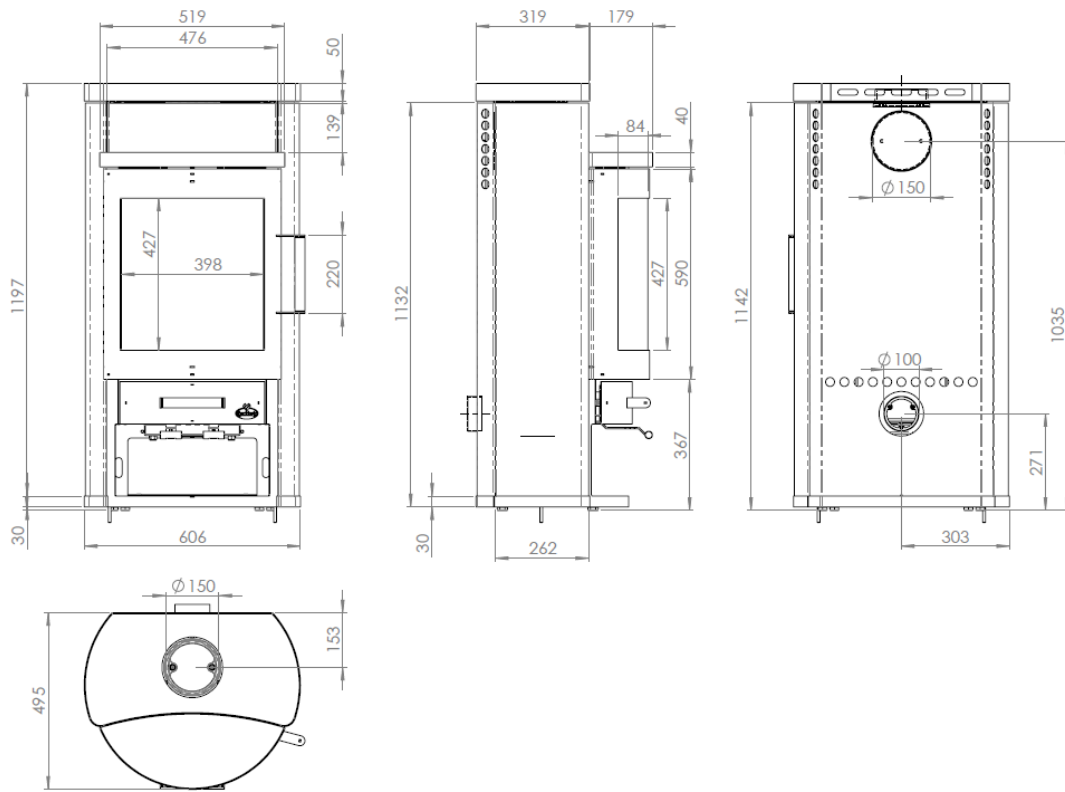
Abbildung 5 - Hauptmaße
