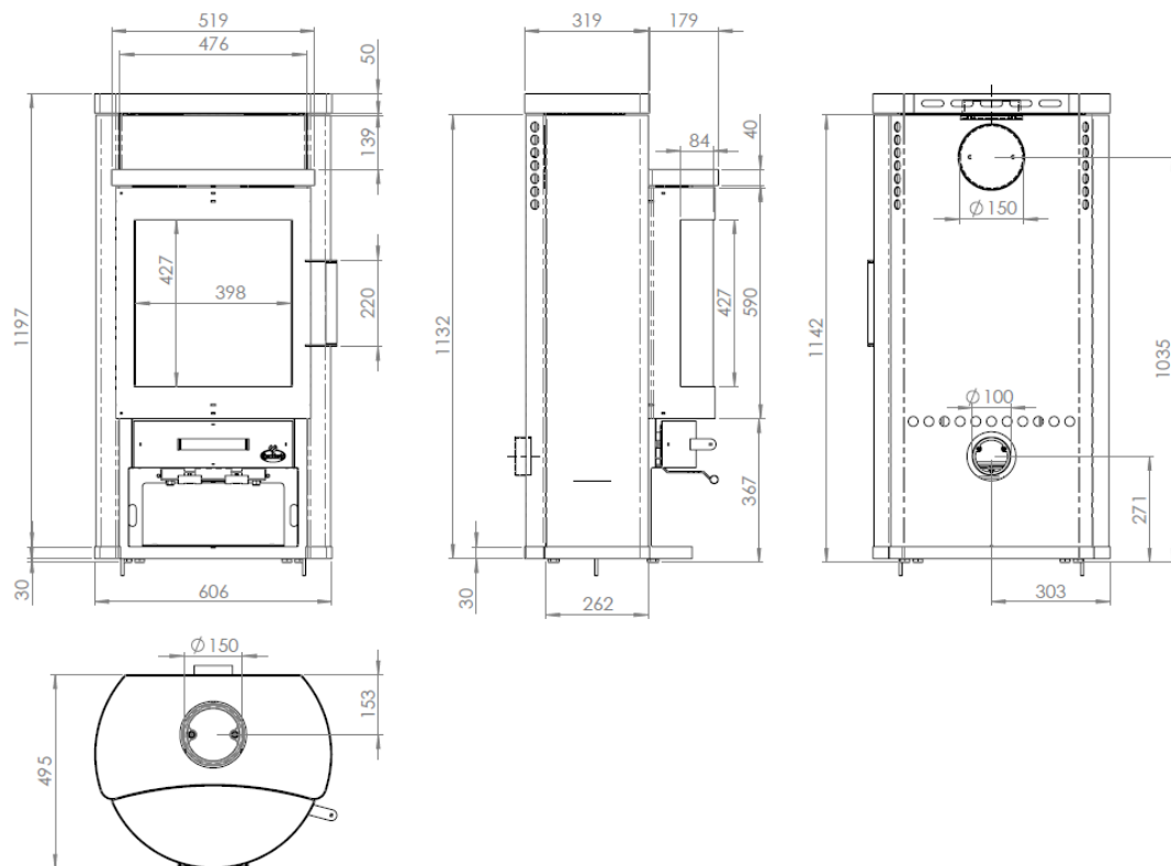
Abbildung 4 - Hauptmaße
