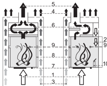
Abbildung 7 – Fire-Plus System, schematische Darstellung
